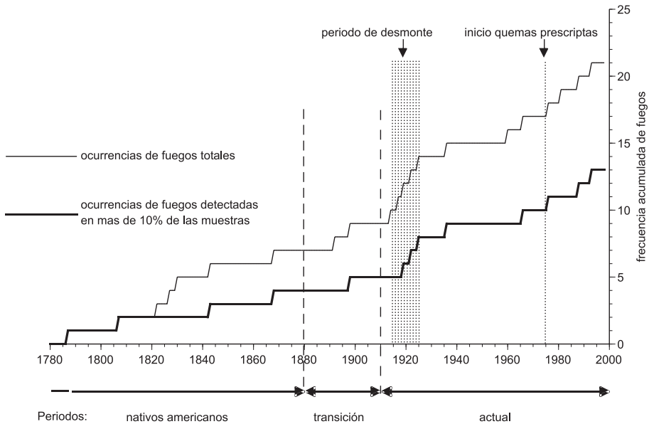
Figura 2. Distribución acumulada de ocurrencias de fuego en el caldenal, estancia La Verde, sur de San Luis Figure 2. Accumulate distribution of fire occurrence in the Caldenal, Estancia La Verde, south of San Luis province
