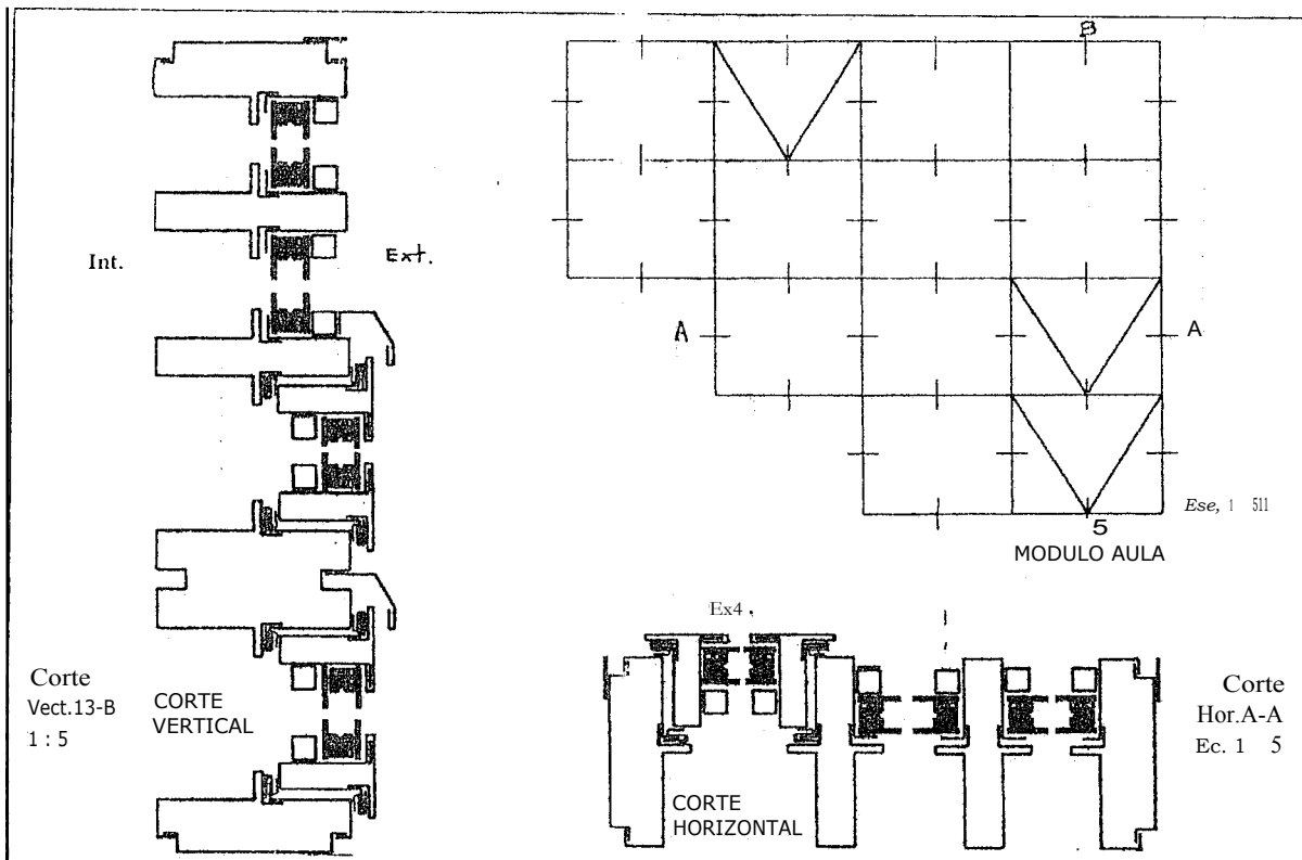
Figura 1. Plano de detalle de carpintería de módulo del aula. Corte vertical y horizontal .
