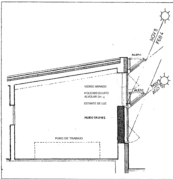
Fig. 5. Meses de sombreado y pleno sol por los aleros.
